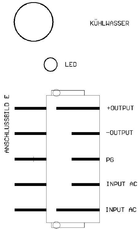
ANSCHLUSSBILD E
