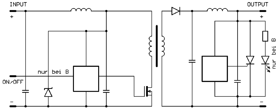
Prinzipschaltbild A+B
