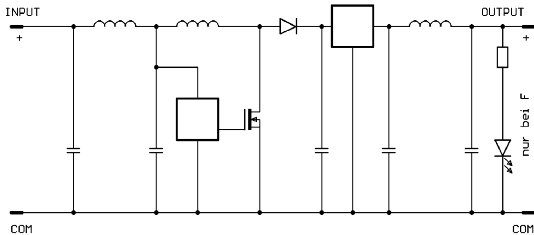
Prinzipschaltbild E+F
