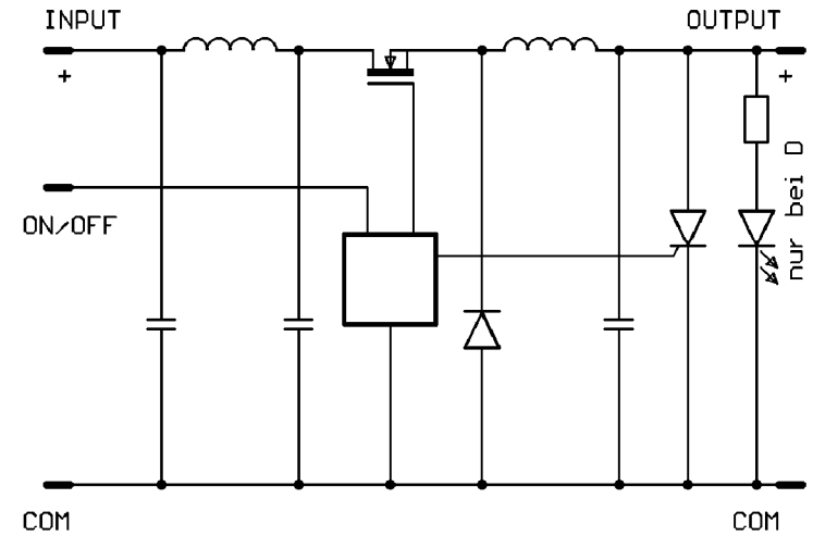
Prinzipschaltbild C+D
