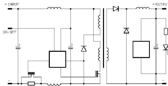
Prinzipschaltbild B
