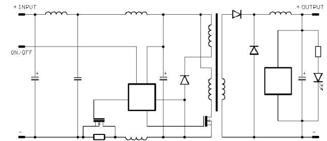
Prinzipschaltbild C
