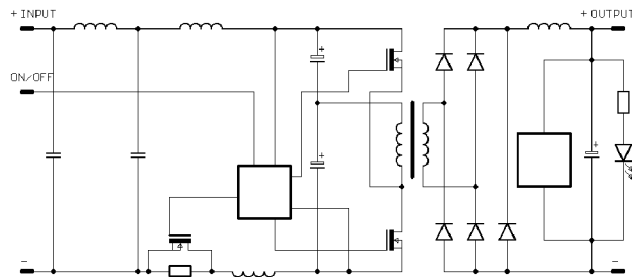
Prinzipschaltbild D
